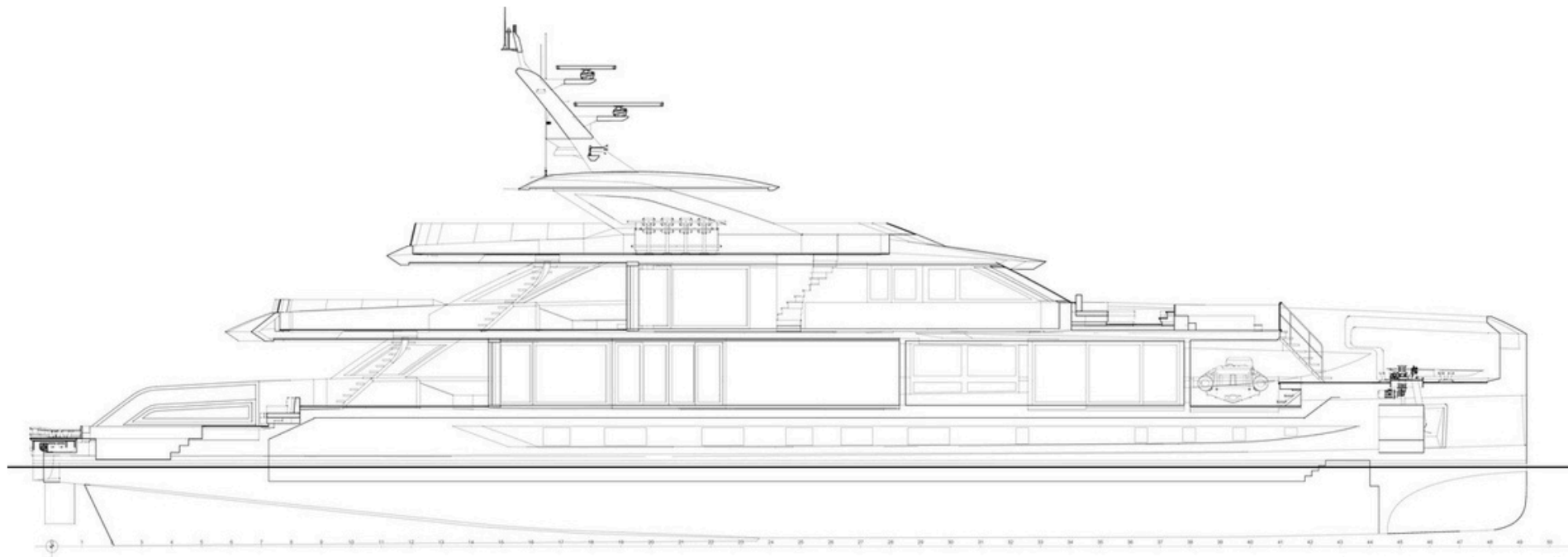
LONGITUDINAL SECTION
